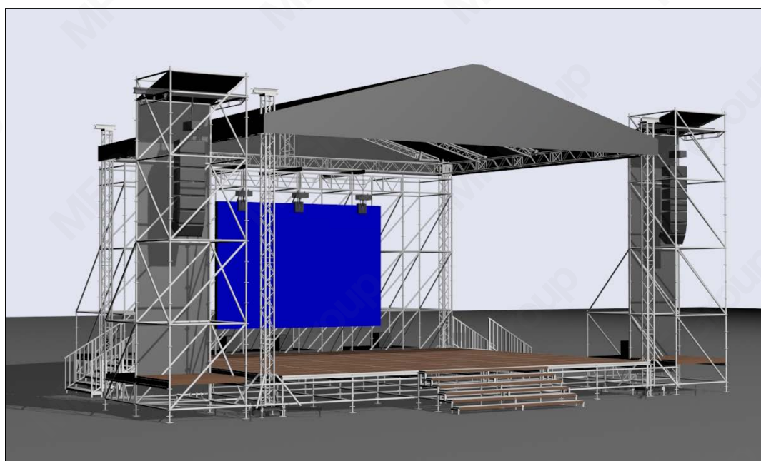
MPT ROOF 12x10 м
