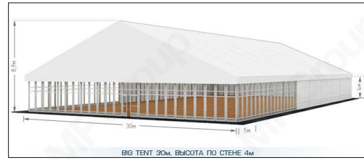
BIG TENT 30м. ВЫСОТА ПО СТЕНЕ 4м
